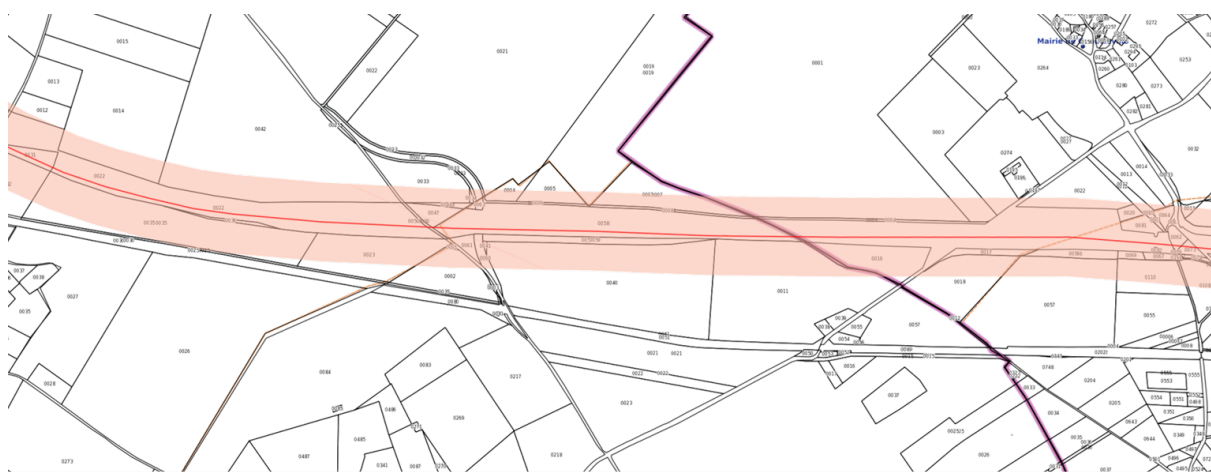
Classement sonore des infrastructures routières et ferroviaires en Seine-Maritime Source DDTM de Seine-Maritime
